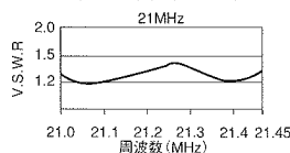
T3-11DX V.S.W.R.特性表
