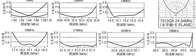
T512GX-T512GX 3040 V.S.W.R.特性表
