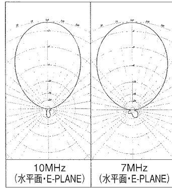
7・10MHz2バンド八木。No-Lossトラップ 採用のハイパワーバージョン。
