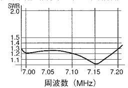
NA-440 V.S.W.R特性表
