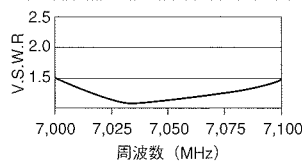
A-240SII V.S.W.R特性表
