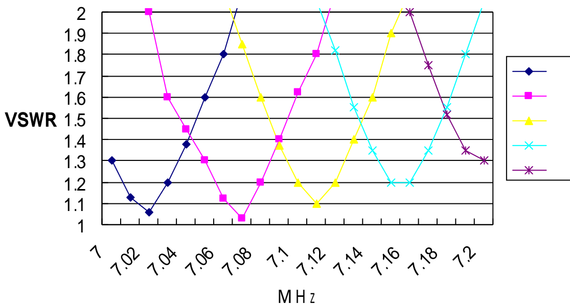
《設置例の VSWR 特性》
