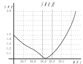
T 2 - 3 V X X の V S W R 特性
